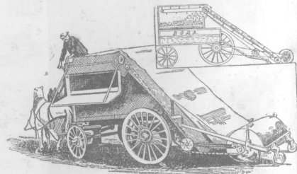
Машина для чистки улицъ.
