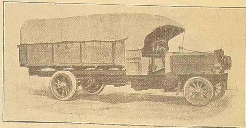
Новый автомобиль германскихъ войскъ сообщенія. — Грузовикъ въ 3' — 4 тоны полезной подъемной силы; можетъ тянуть еще прицепной вагонъ съ грузомъ въ 2—2½ тонны. Скорость 4—16 километровъ въ часъ. Дальность пробѣга до 250 километровъ.
