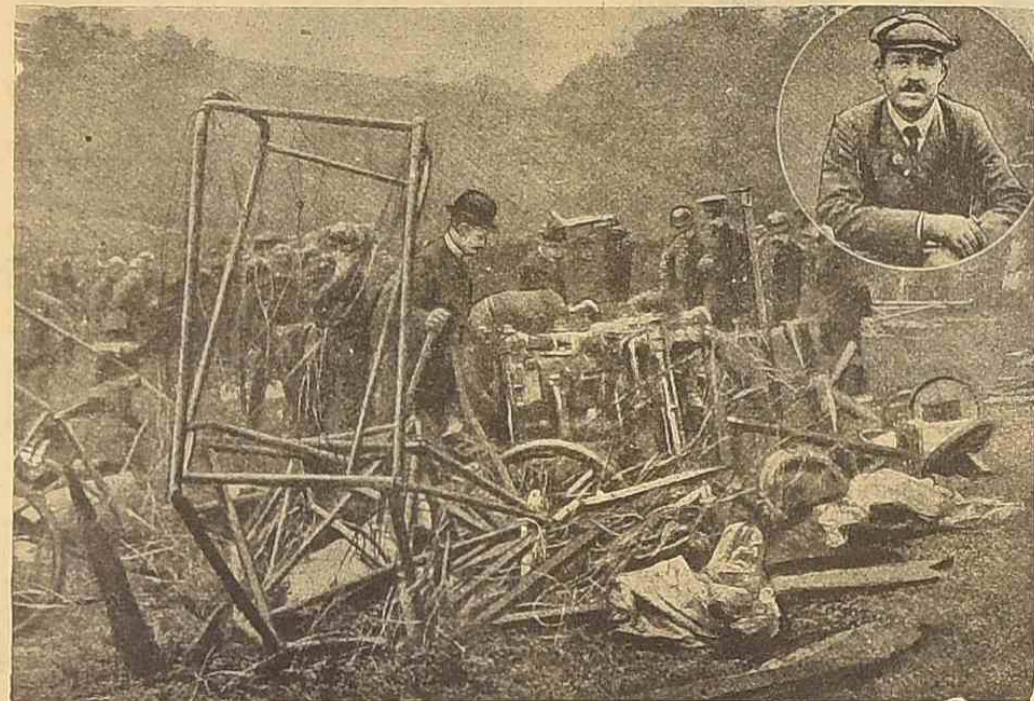
Крушение дирижабля „Зрблз“ у Лейхлингена (Германія). Сверху портретъ строителя дирижабля Эрблз, погибшаго при крушеніи.
