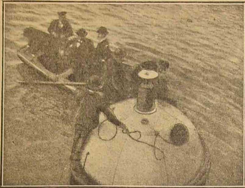
Металлическій буй новой системы (Д нвинга) для спасанія потерѣвшихъ кор. блекрушеніе — для 16 человекъ.
