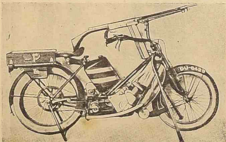
Мотоциклетка для военныхъ цѣлей. Мотоциклетка съ ружьемъ, выстрѣляющая на Лондонской выставкѣ. Ружье дѣлаетъ 300 выстрѣловъ въ минуту.
